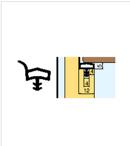
Joint de porte K3231
