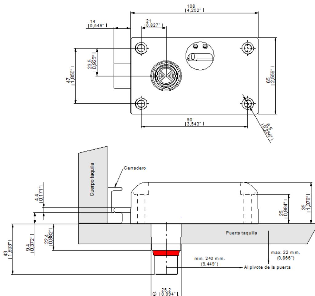
Illustration 2. Dimensions de la serrure OTS 20 Batteryless en mm. (Pouces).
